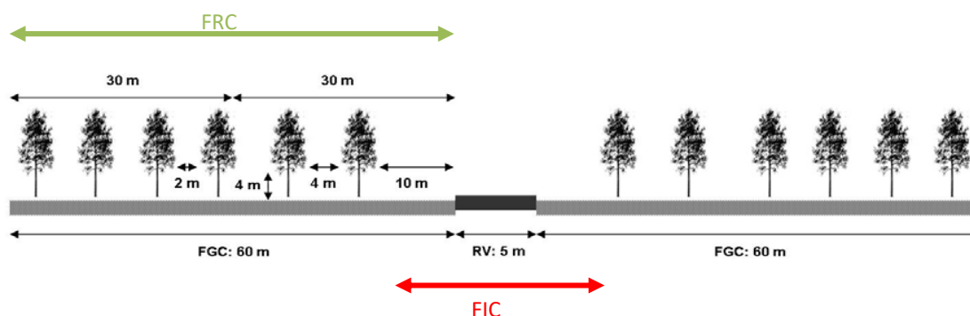
Figura 2 - Secção transversal do modelo da RPFGC.
