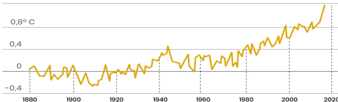
Gráfico 24 - Variação da temperatura média entre 1880 e 2014.
