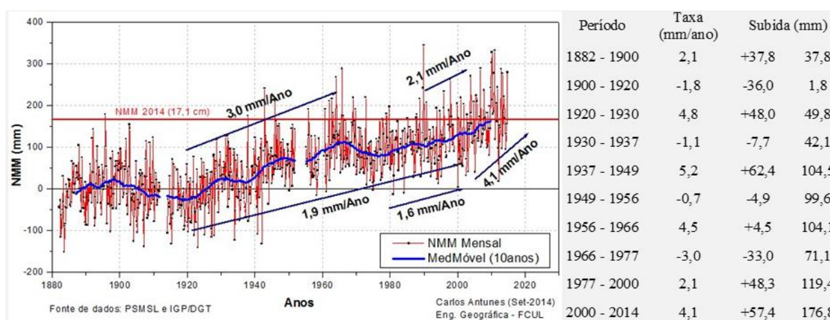
Gráfico 25 - Variação do nível médio do mar (NMM), entre 1880 e 2014.
